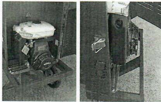
Fig. 2.3. Montaje del motor de explosión
