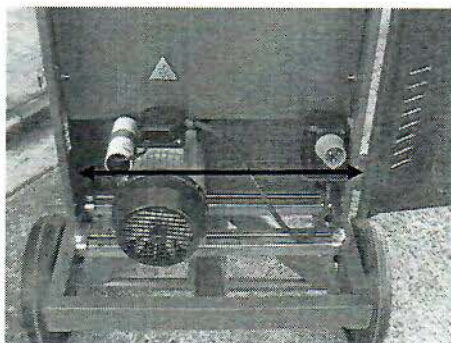
Fig. 5.2. Desplazamiento para tensado de correas
