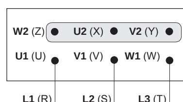
Y Connection
