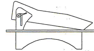
USO DE LA MESA REGULABLE: LA PROTECCIÓN SE FIJA EN LO ALTO DE LA GUÍA
