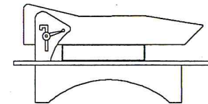
CORTE DEL MATERIAL: EL DISCO QUEDA TOTALMENTE PROTEGIDO
