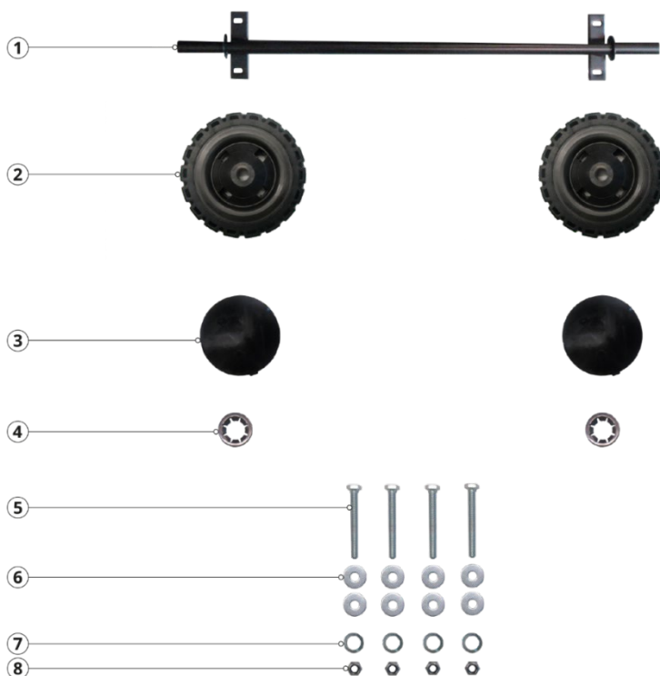
Imagen 21: Lista de materiales del Kit 2: Eje y ruedas.
