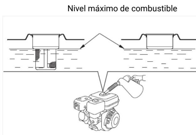
Imagen 10: Nivel máximo de combustible.
