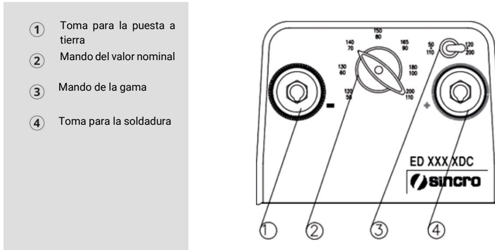
Imagen 17: Descripción del panel de la motosoldadora DGH 220 W DC.
